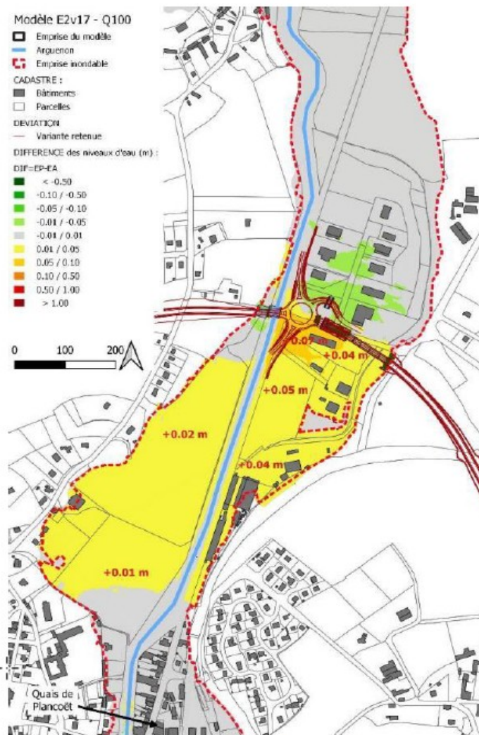
Différence des niveaux d'eau modélisés entre l'état projet et l'état initial - Modèle E2v17 - Q100
