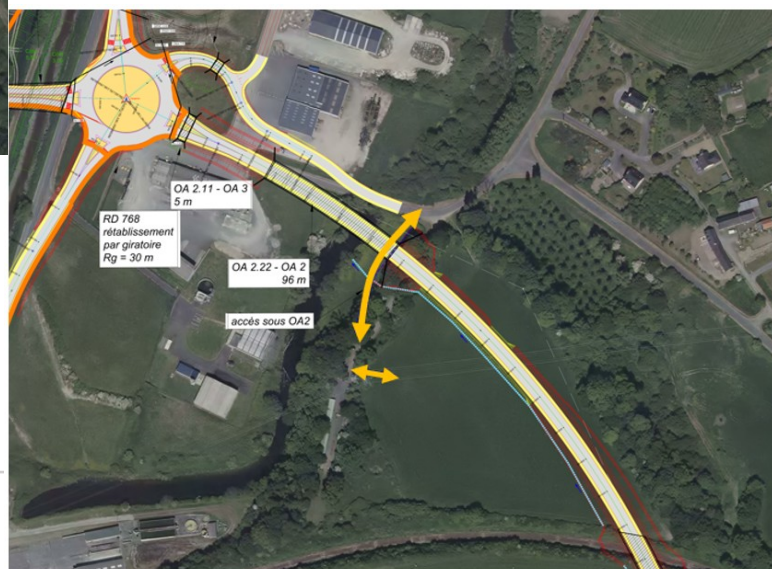
Variante B : élargissement OA2
