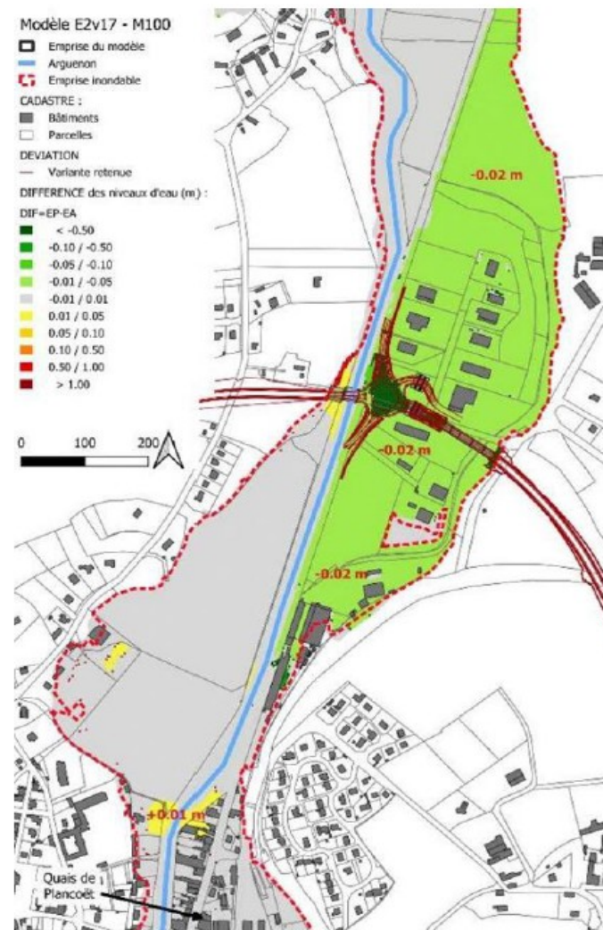
Différence des niveaux d'eau modélisés entre l'état projet et l'état initial - Modèle E2v17 - M100
