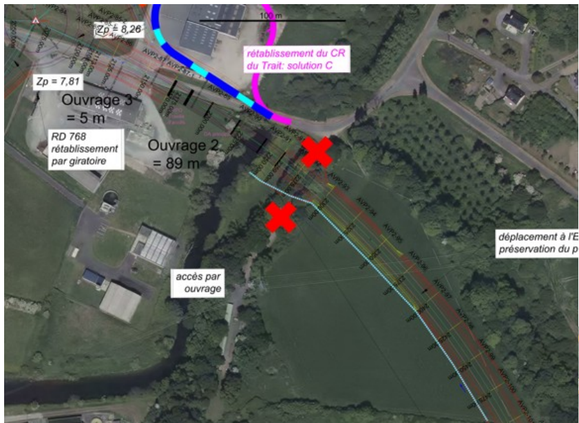
Variante A : pas de rétablissement de l'accès
