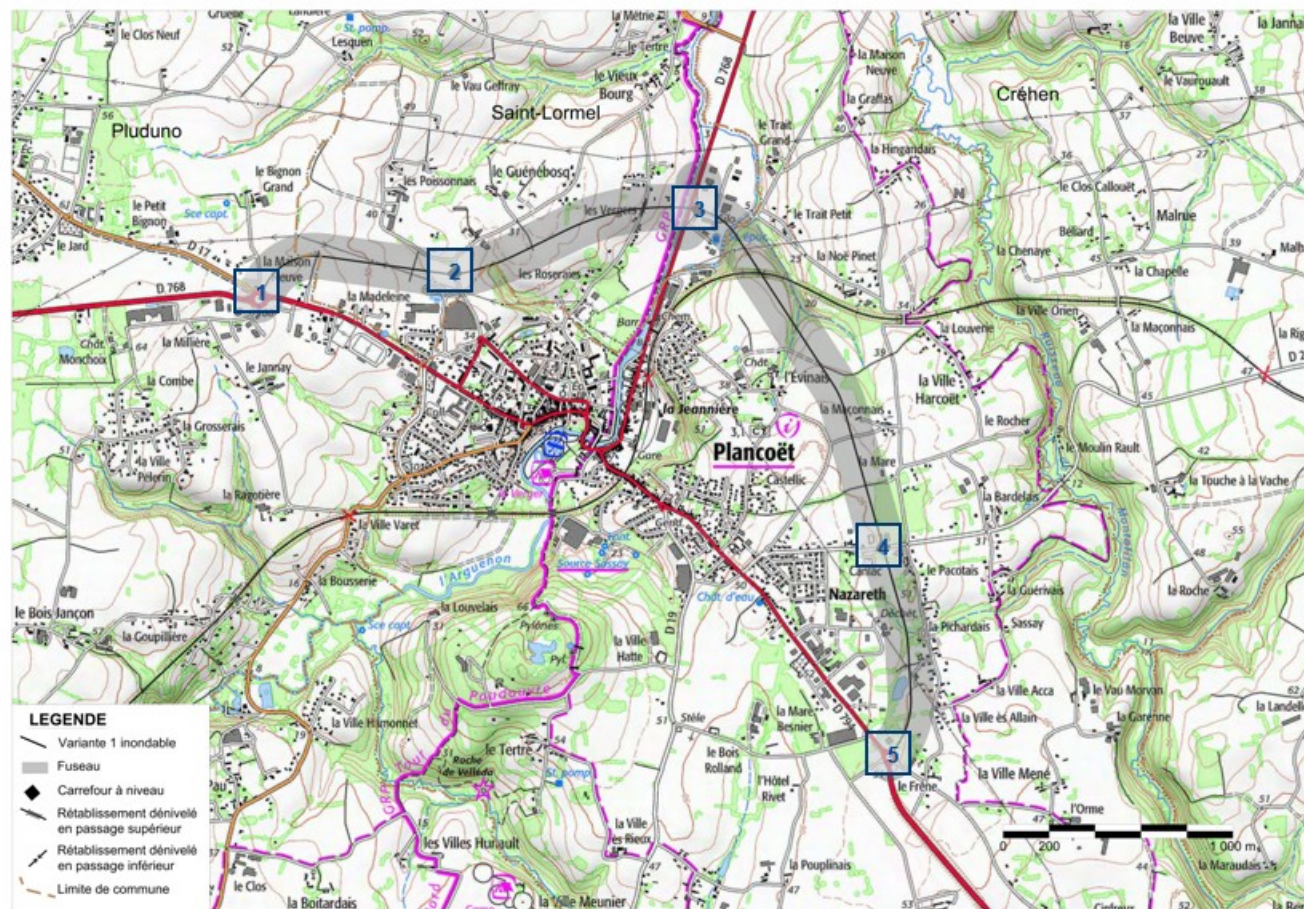
Localisation des points d'échanges
