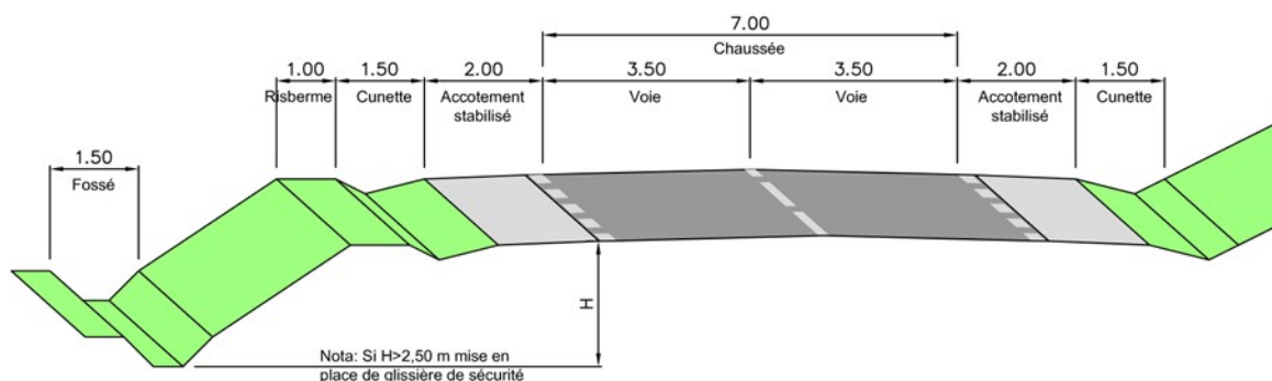
Profil en travers type de la voirie
